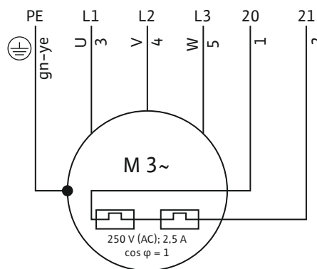
Fig. 7: Schéma zapojení 3~ motoru
